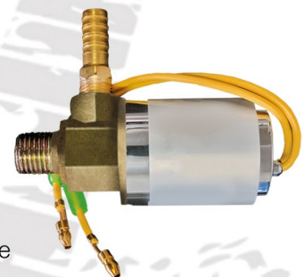
VS-106 - Válvula solenóide buzina bivolt
